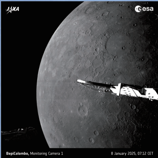
©ESA/BepiColombo/MTM
